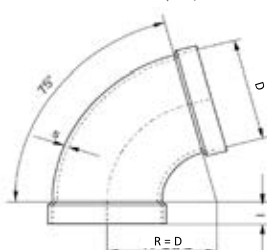
XX.DDD.L.0030 / \zeta = 0,10
