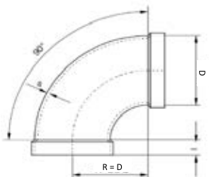
XX.DDD.L.0045 / \zeta = 0,15
