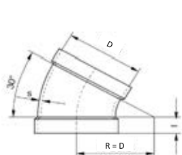
XX.DDD.L.0030 / \zeta = 0,10
