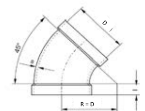
XX.DDD.L.0045 / \zeta = 0,15
