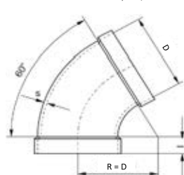
XX.DDD.L.0015 / \zeta = 0,05
