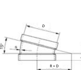
XX.DDD.L.0015 / \zeta = 0,05
