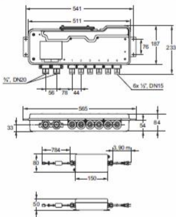
Rysunek wymiarowy
